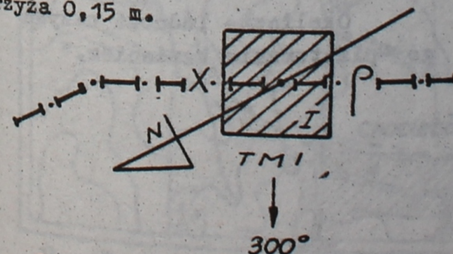
Rys.12. Orientacja słupa I.
