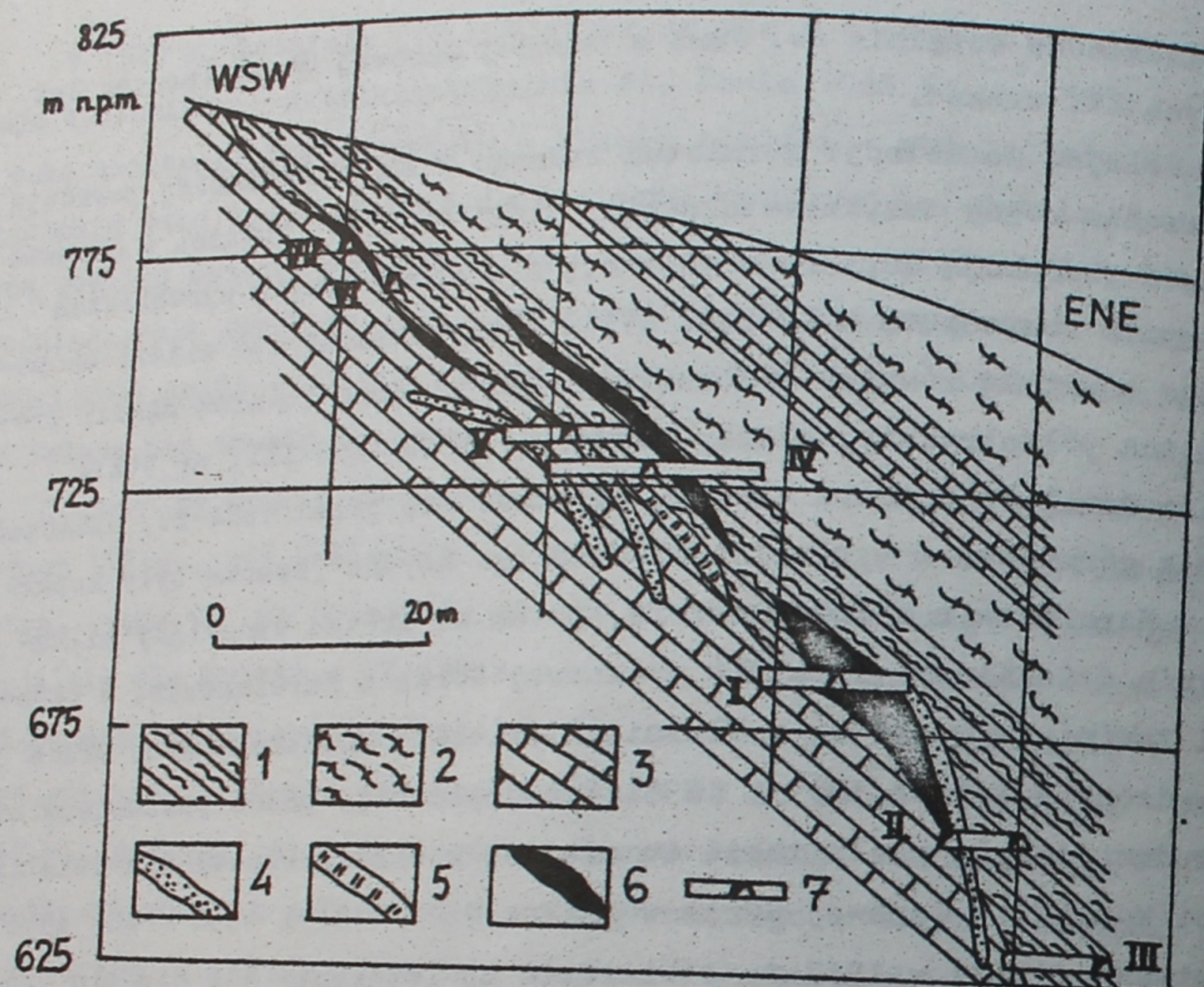
Rys.1. Przekrój geologiczny przez strefę zmineralizowaną w Kletnie (wg Banasia 1965)
